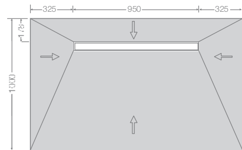
4-seitiges Gefälle
